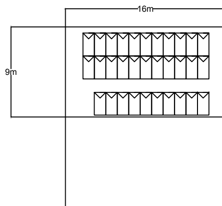
PRÉDIO 2 2 FILEIRAS DE 11 MÓDULOS 1 FILEIRA DE 10 MÓDULOS
